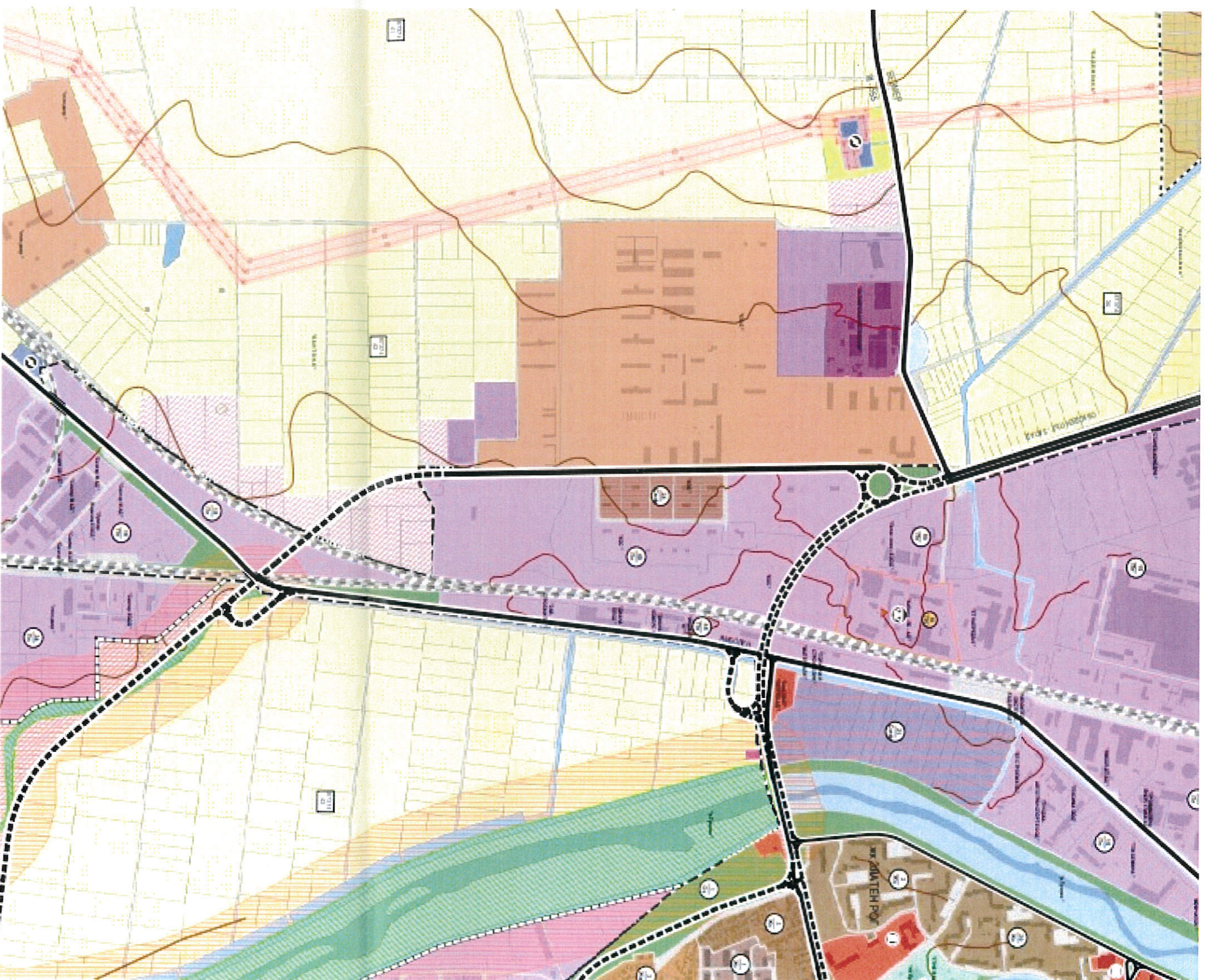
ИЗВАДКА ОТ ДЕЙСТВАЩИЯ ОБЩ УСТРОЙСТВЕН ПЛАН НА ОБЩИНА ЯМБОЛ М 1:10000
