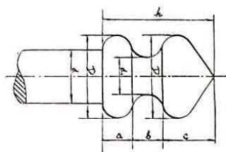
Фиг. 4 Накрайник за напречник
