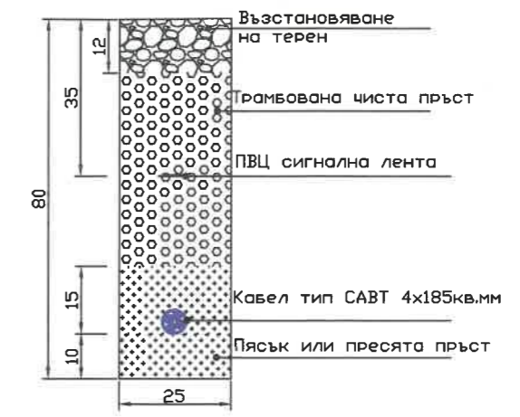
ДЕТАЙЛ -1
